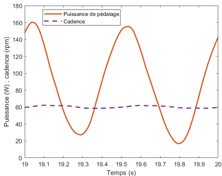
Fig 1 : Exemple typique de puissance utilisateur sur une génératrice GénéPi
